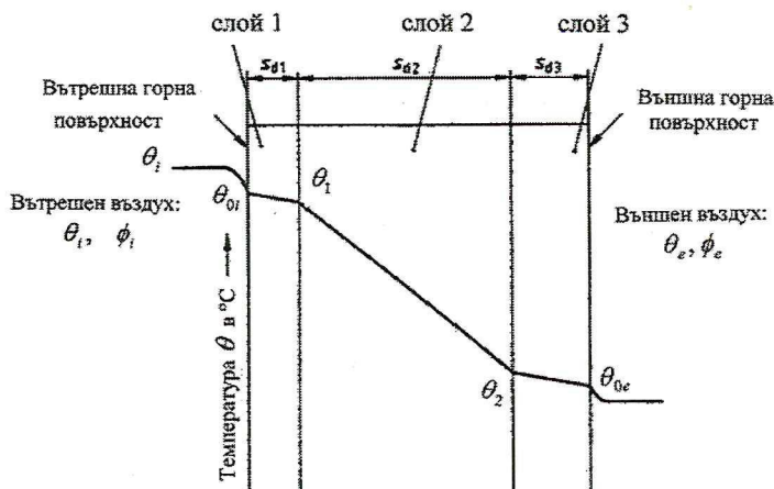
фиг. 6.1. Схема на кривата на температурното разпределение
