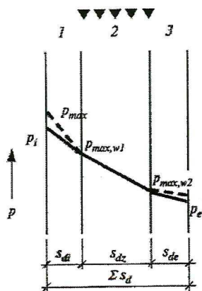
Фиг. 6.5а. Дифузия на водната пара с кондензационен пад във вътрешността на ограждащата конструкция или елемент
